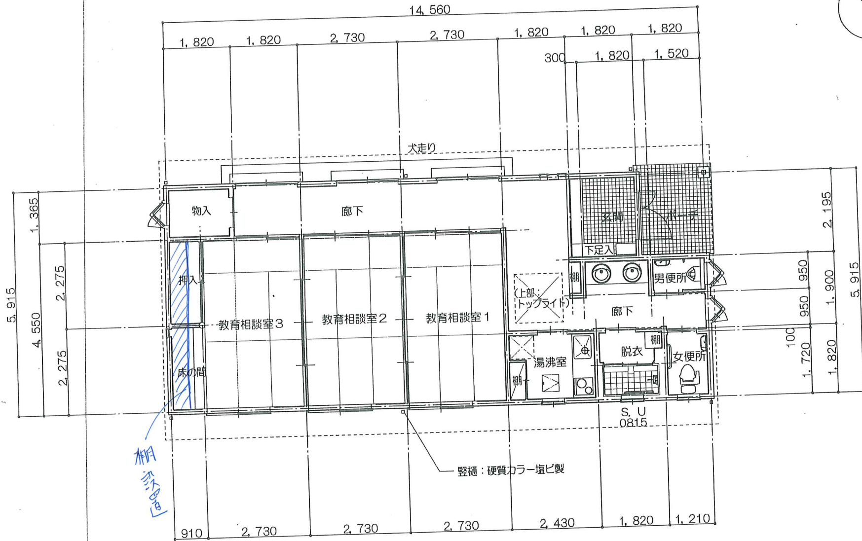
1階平面図 1/100
