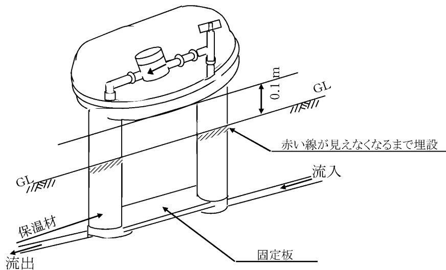
地上式メータユニット
