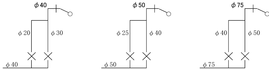
図 4 間接排水構造標準図
