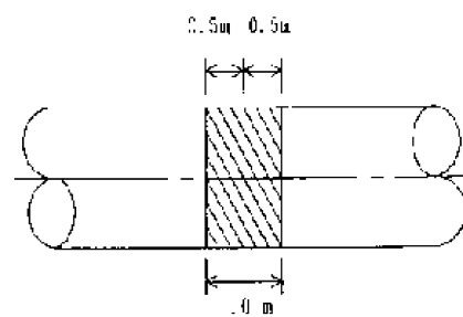
直部の重ね継手詳細
