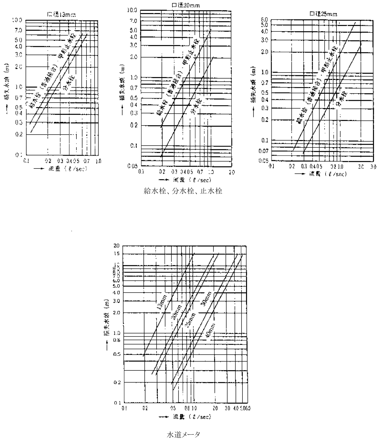
図 3-3-3 水栓類、水道メータ等の損失水頭
